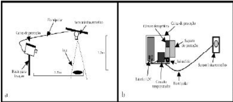
Figura 2. (a) Esquema do sistema de câmara fotográfica com sensor infravermelho disposto no campo (adaptado de Rittl, 1998) e (b) Esquema dos compartimentos internos do dispositivo fotográfico.
